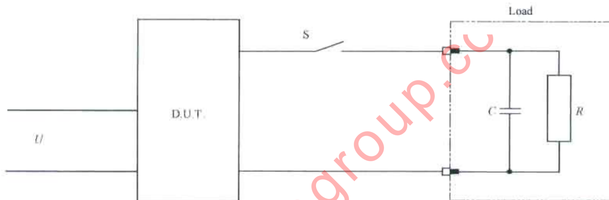
a) 启动过程中的电流测量线路
