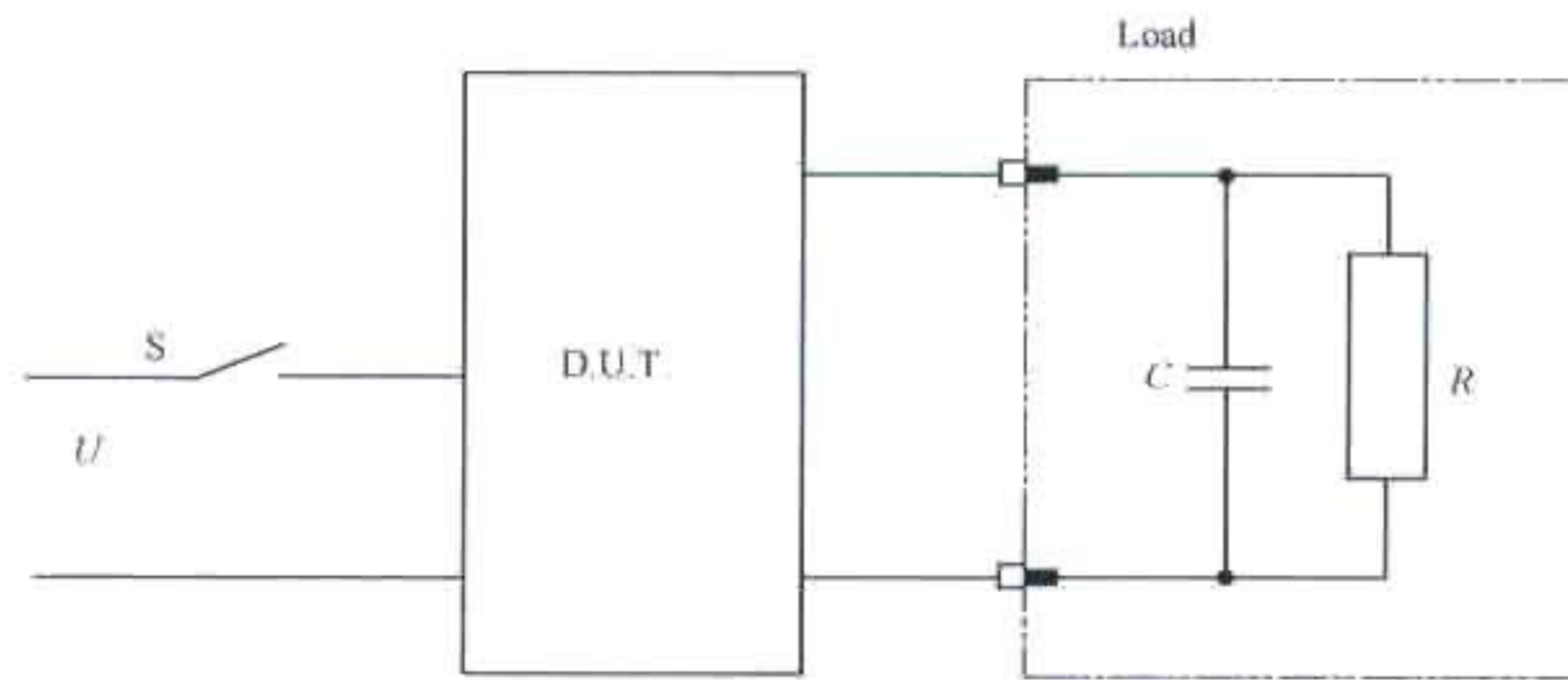
a) 启动过程中的电流测量线路
