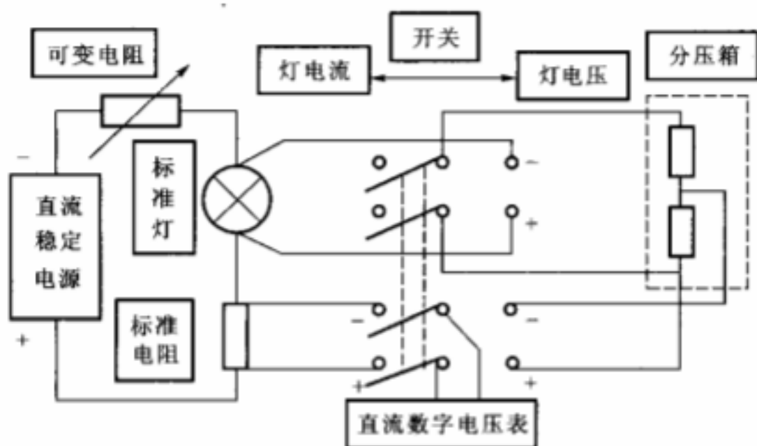
图3 直流供电的电测线路图
